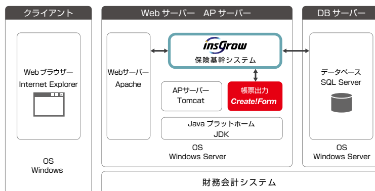
InsGrowのシステム図
